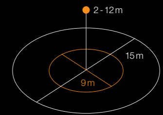
Montagehöhe 2 - 12 m True Presence®-Bereich Ø 9 м / 64 м² Präsenzbereich Ø 15 м / 177 м²
